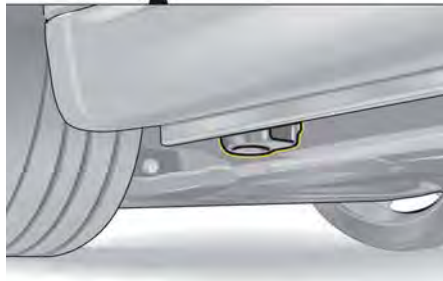
フロント側のリフティング・プラットフォームおよびジャッキ用のジャッキ・ポイント
