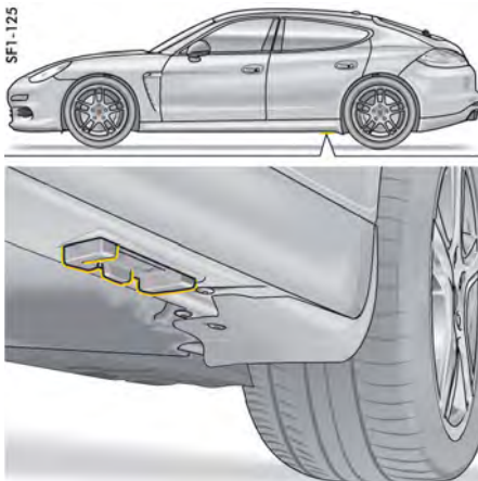
リア側のリフティング・プラットフォームとジャッキ用のジャッキ・ポイント
