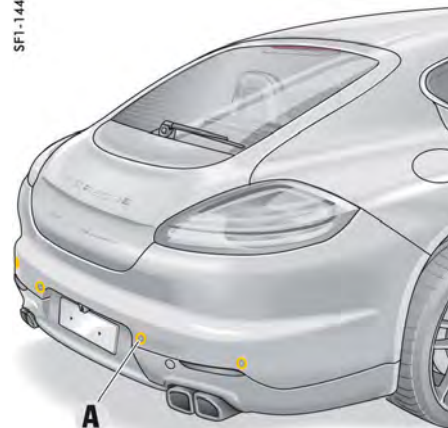
リヤ超音波センサー
