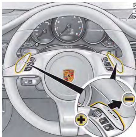
シフト・ボタン付きステアリング・ホイール
