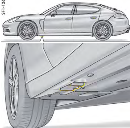
フロント側のリフティング・プラットフォームとジャッキ用のジャッキ・ポイント
