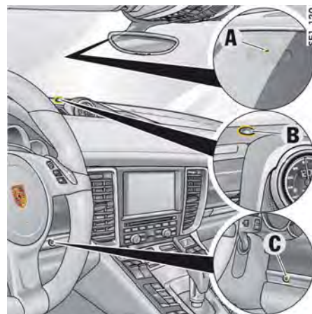
A - 結露センサー
