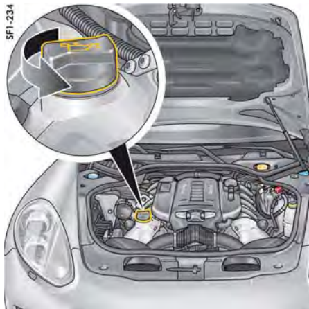
エンジン・オイルの給油口 (Panamera S E-Hybrid、Panameraディーゼル*を除く)
