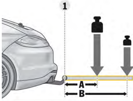
アタッチメントおよびアクセサリ負荷配分図
